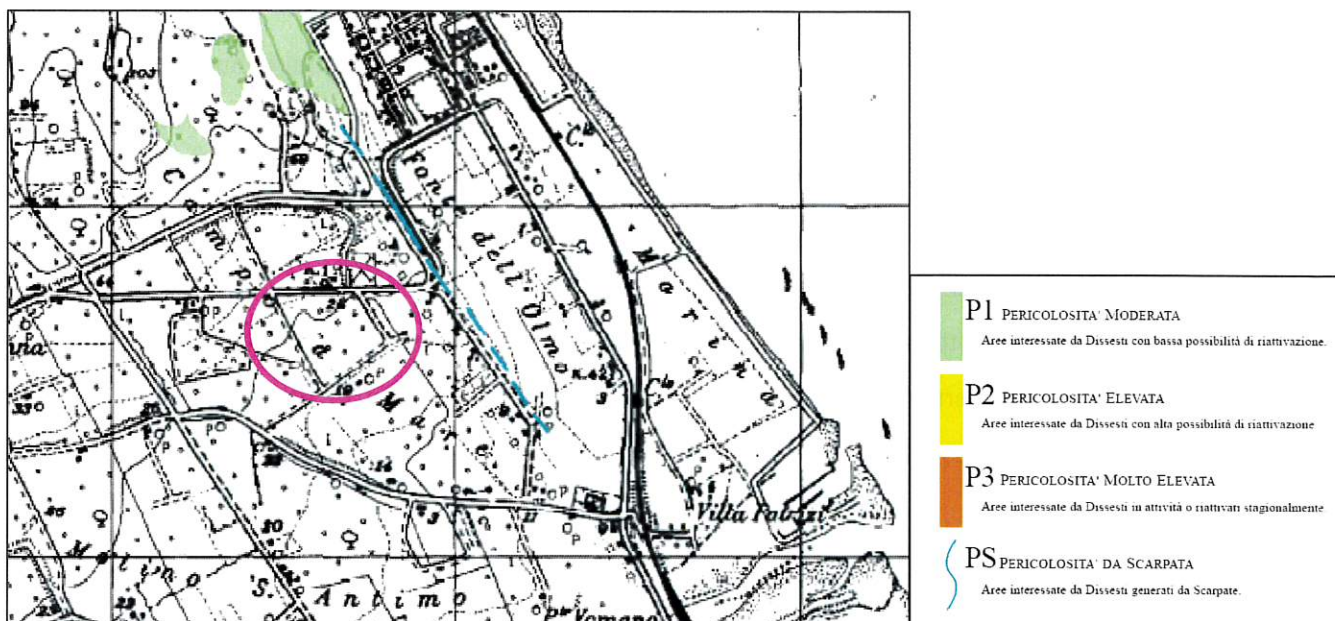
Figura 5: PIANO STRALCIO DI BACINO PER L'ASSETTO IDROGEOLOGICO "FENOMENI GRAVITATIVI E PROCESSI EROSIVI" REDATTO DALLA REGIONE ABRUZZO - CARTA DELLA PERICOLOSITÀ - TAVOLA 340 O
